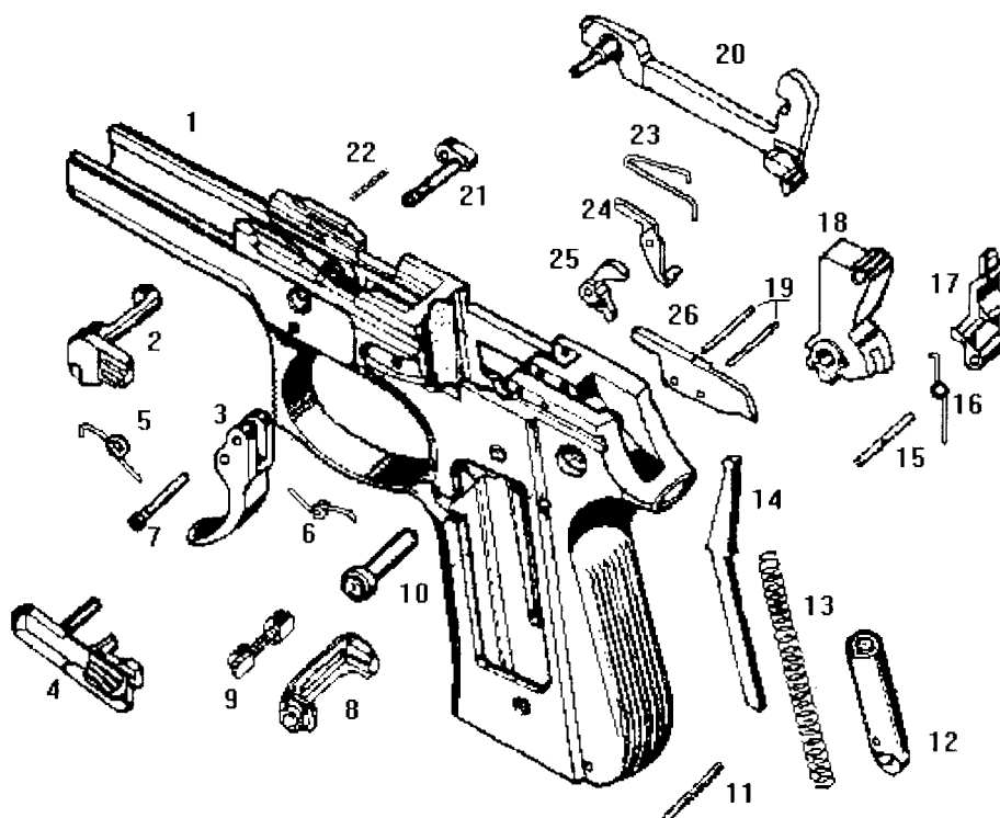
FUSTO Mod. 92 F (esploso delle parti)
