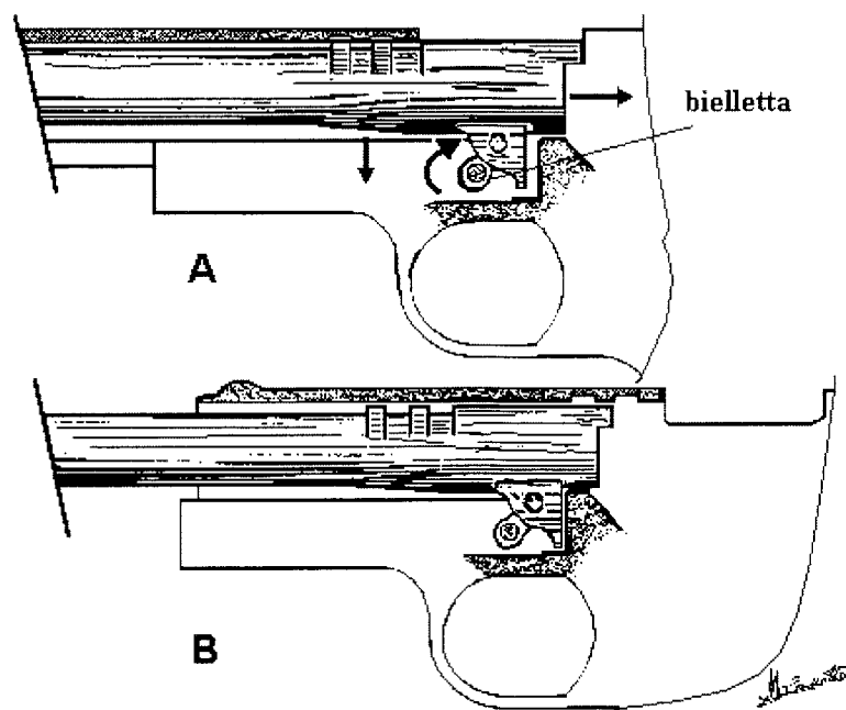
Disegno schematico di chiusura geometrica, a corto rinculo di canna, sistema "Browning"
